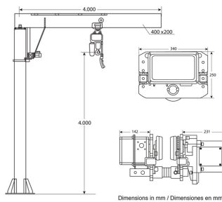
Dimensions in mm / Dimensiones en mm
